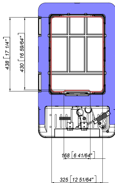
Sezione F-F
