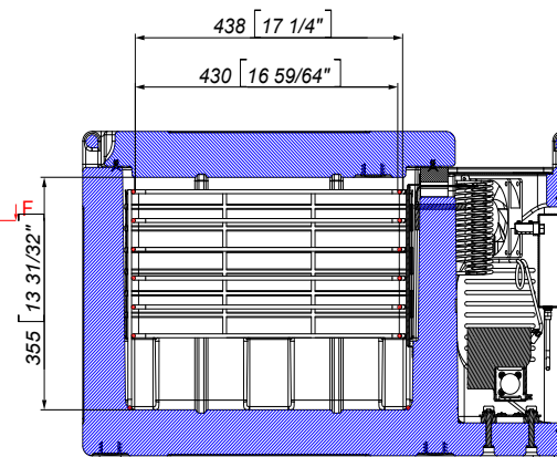
Sezione E-E
