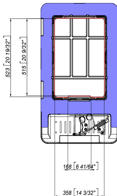
Sezione F-F
