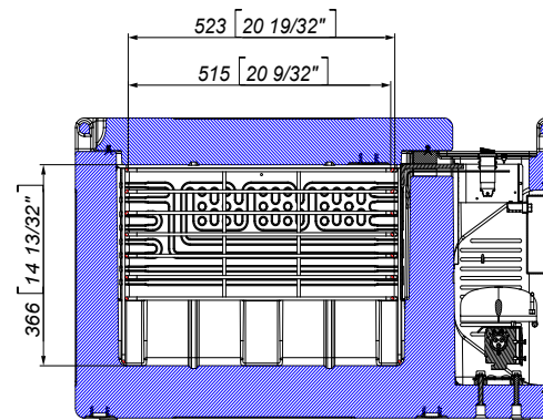
Sezione E-E
