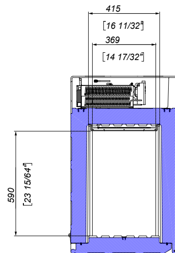
Sezione F-F
