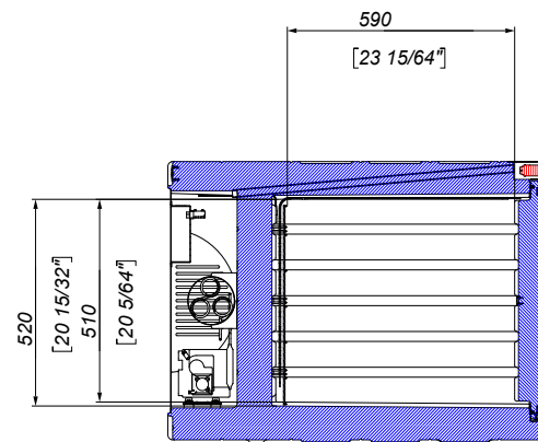
Sezione E-E
