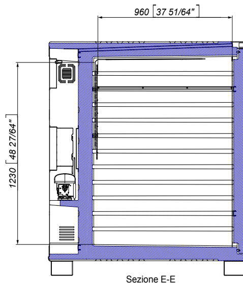
Sezione E-E
