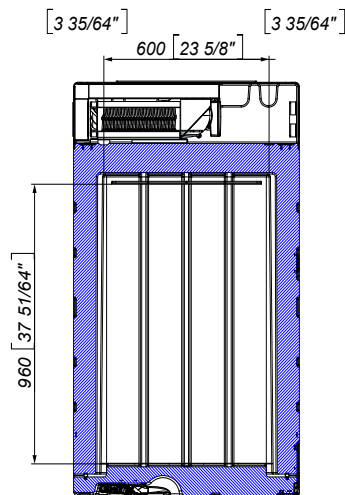
Sezione F-F
